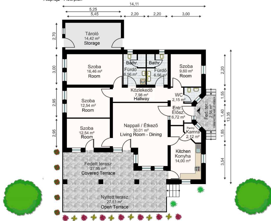
Alaprajz - Floorplan
